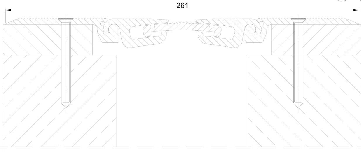
CONECTO AL 125.20.N SECTION
