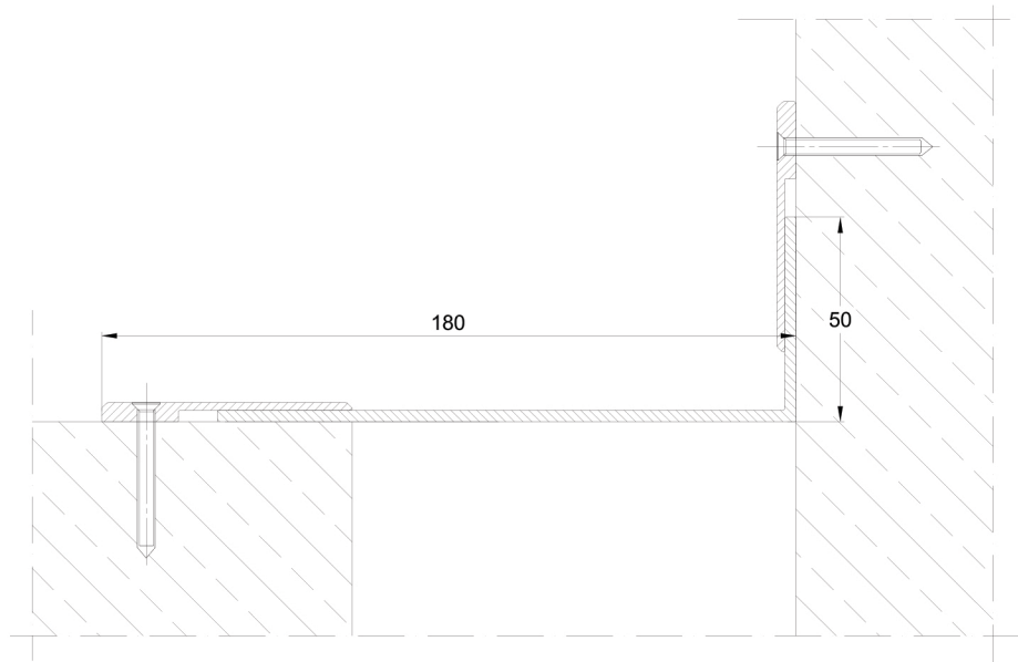
CONECTO WA 260 CV SECTION
